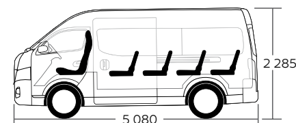
Carroçaria Alargada, Tejadilho Alto Alargado Carroçaria Alargada, Tejadilho Alto
